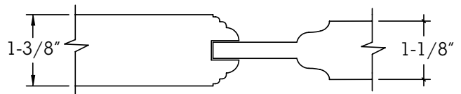
Interior Door Profile H8A
