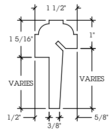
AS4 - KERFED ASTRAGAL
