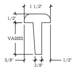
AS3 - NONKERFED ASTRAGAL
