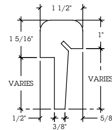
AS1 - KERFED ASTRAGAL
