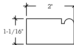
B3 BRICKMOULD
