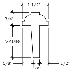
AS6 - NONKERFED ASTRAGAL
